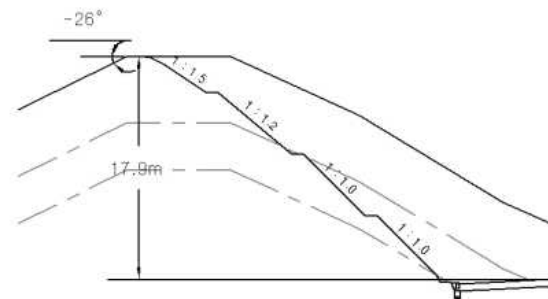
<A-A'단면>
